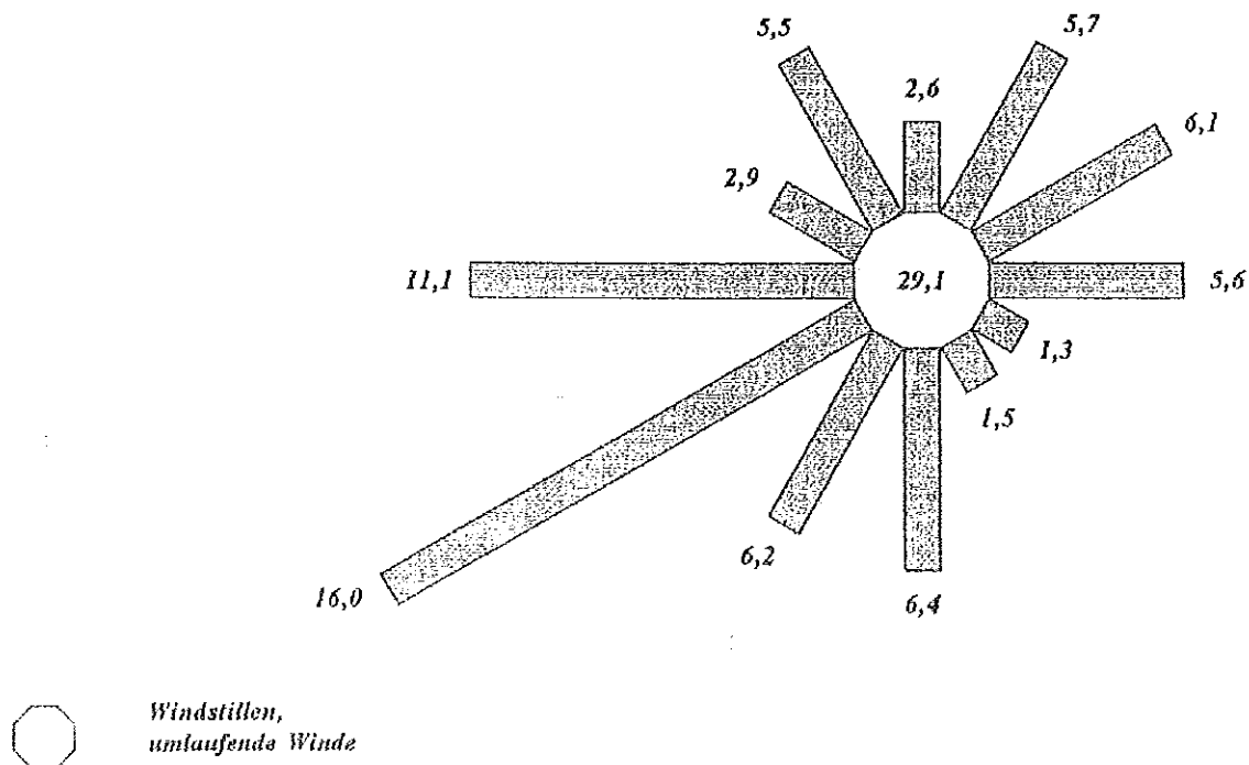
Abbildung: Windrichtungsverteilung für den Winter, Meßstelle Salzelmen. Sinngemäß übertragbar auf Standort IPW. Quelle: Gutachten des Deutschen Wetterdienstes für Schönebeck, 1997.
