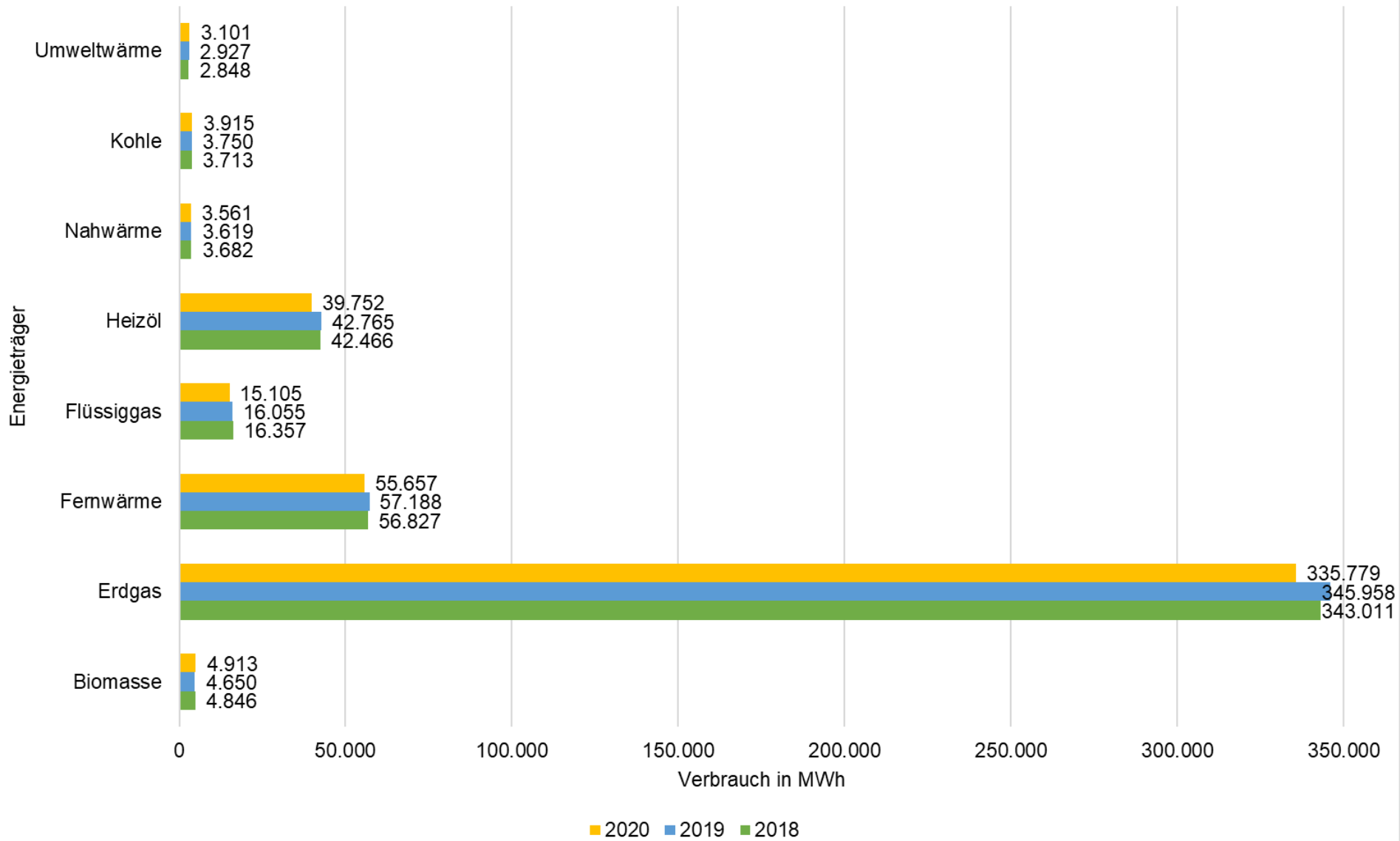
Wärmeerzeugung nach Energieträger
