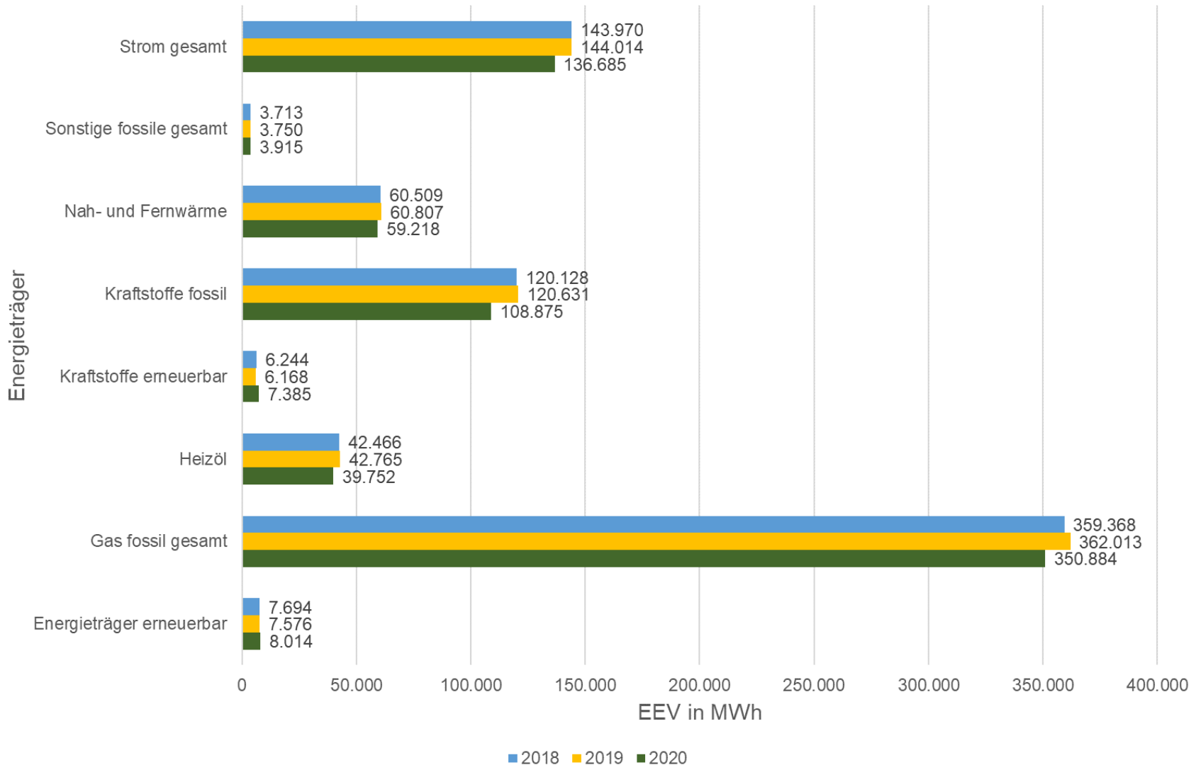
Endenergieverbrauch nach Energieträgern
